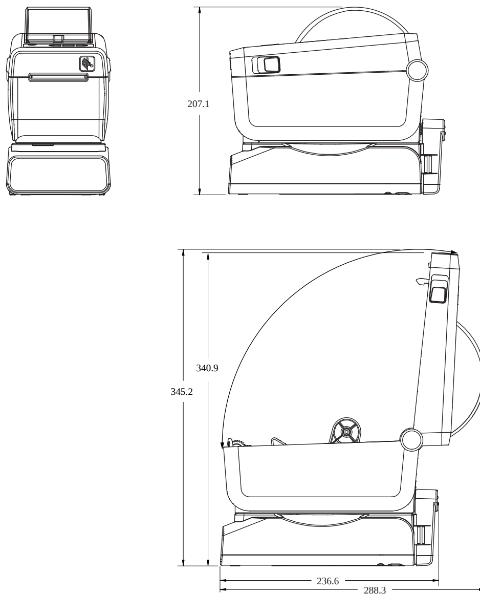
図 19 ZD411D プリンタ (一体型バッテリー ベース オプション付き)
