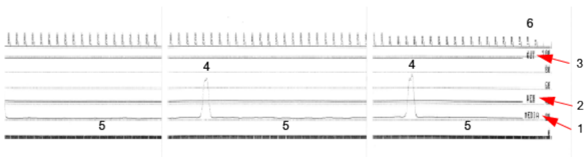
図 10 センサー プロフィール (ギャップ/ウェブ用紙)
