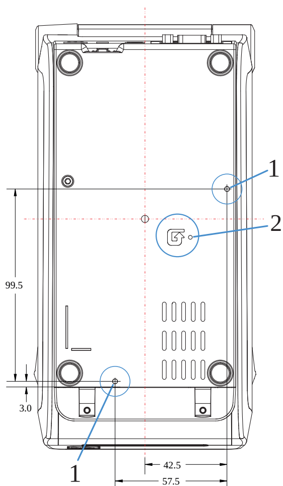
図 20 ZD411D 標準取り付け
