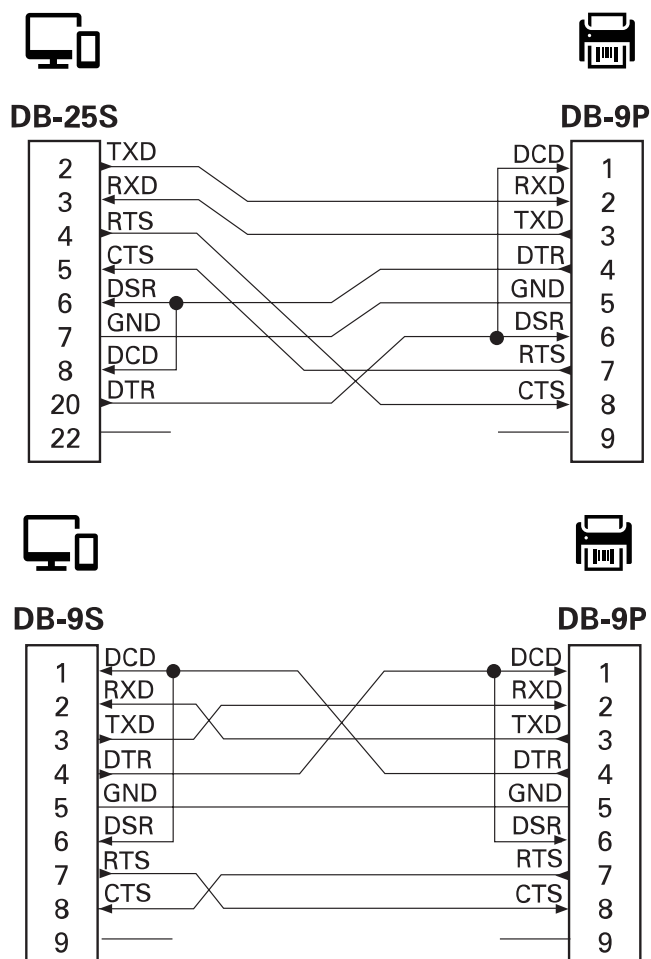
図 14 プリンタを DTE デバイスに接続
