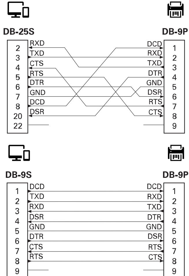
図 15 プリンタを DCE デバイスに接続
