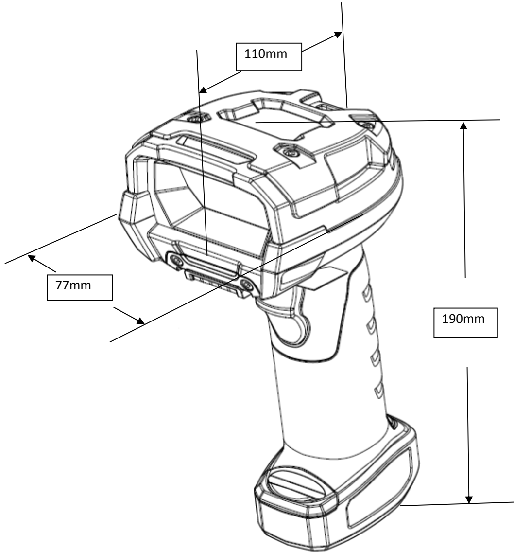
DS3678 外形寸法図
