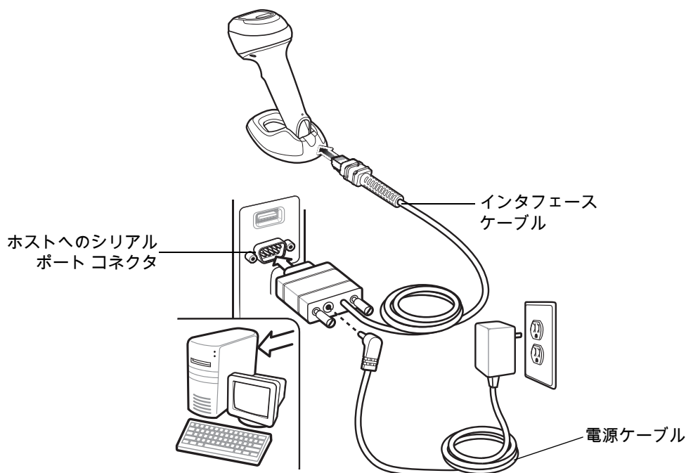
図 16 RS-232 接続
