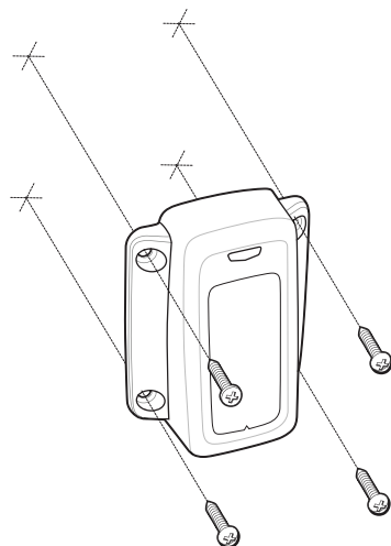
図 B-13 壁面取り付けドングル
